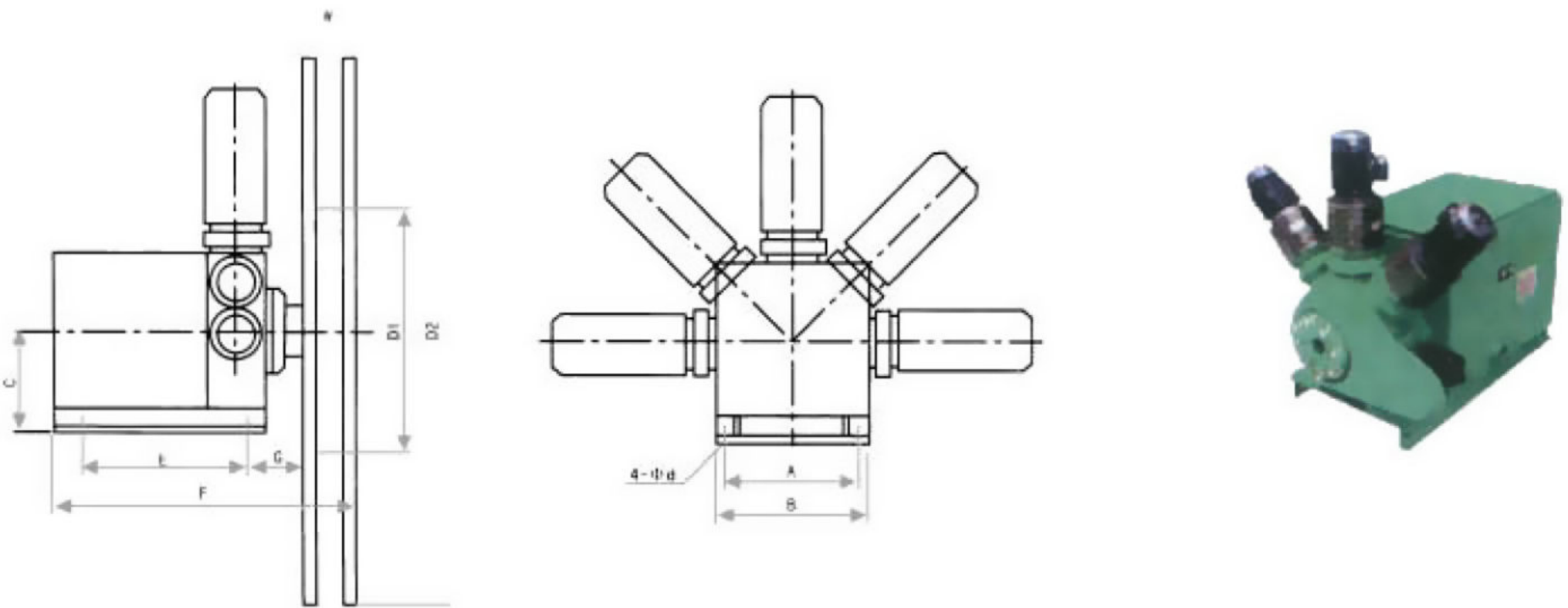
外形尺寸图 Dimensions Figure
