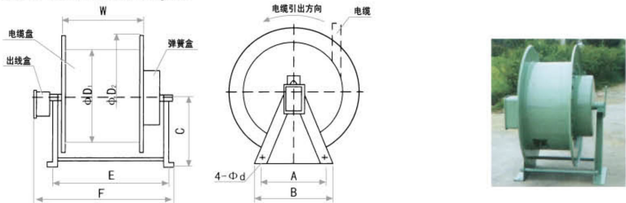
外形尺寸图 Dimensions Figure
