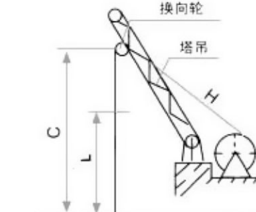
方式B垂直经换向轮卷取
