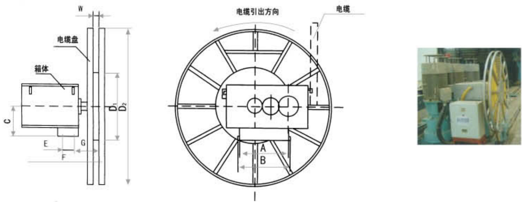
主要技术参数 Main technical data
