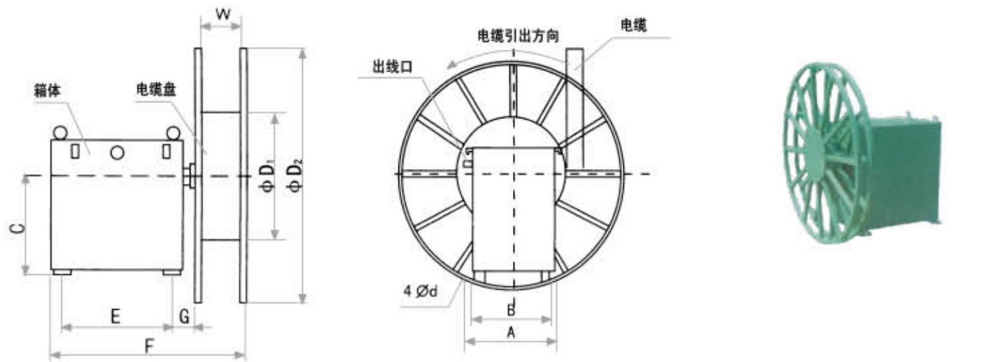
外形尺寸图 Dimensions Figure
