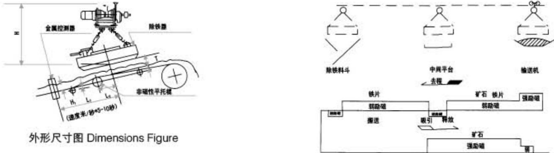
注：L1、L2根据除铁器型号不同而取不同的值。H1、一般取100~120mm。 工作原理示意图 Schematic diagram of
